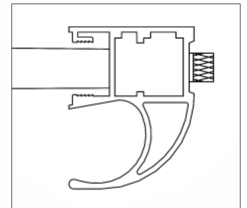
C-FRAME
